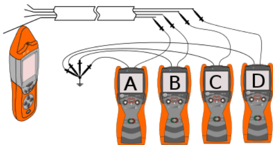
Obr. 38 Identifikace žil ve vodiči – režim U
