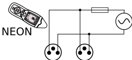
Obr. 14 Schéma režimu vyhledávání elektrického pole 50Hz/60Hz.
