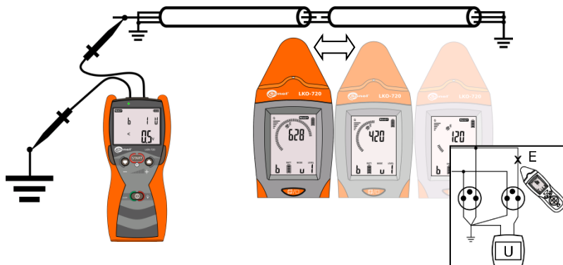
Obr. 26 Lokalizace přerušení
