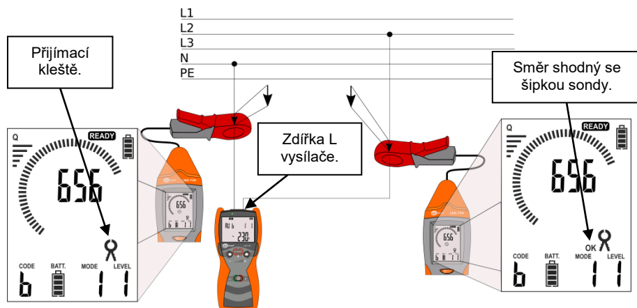
Obr. 40 Příjemcí kleště – vynucení proudu v lokalizovaném obvodu
